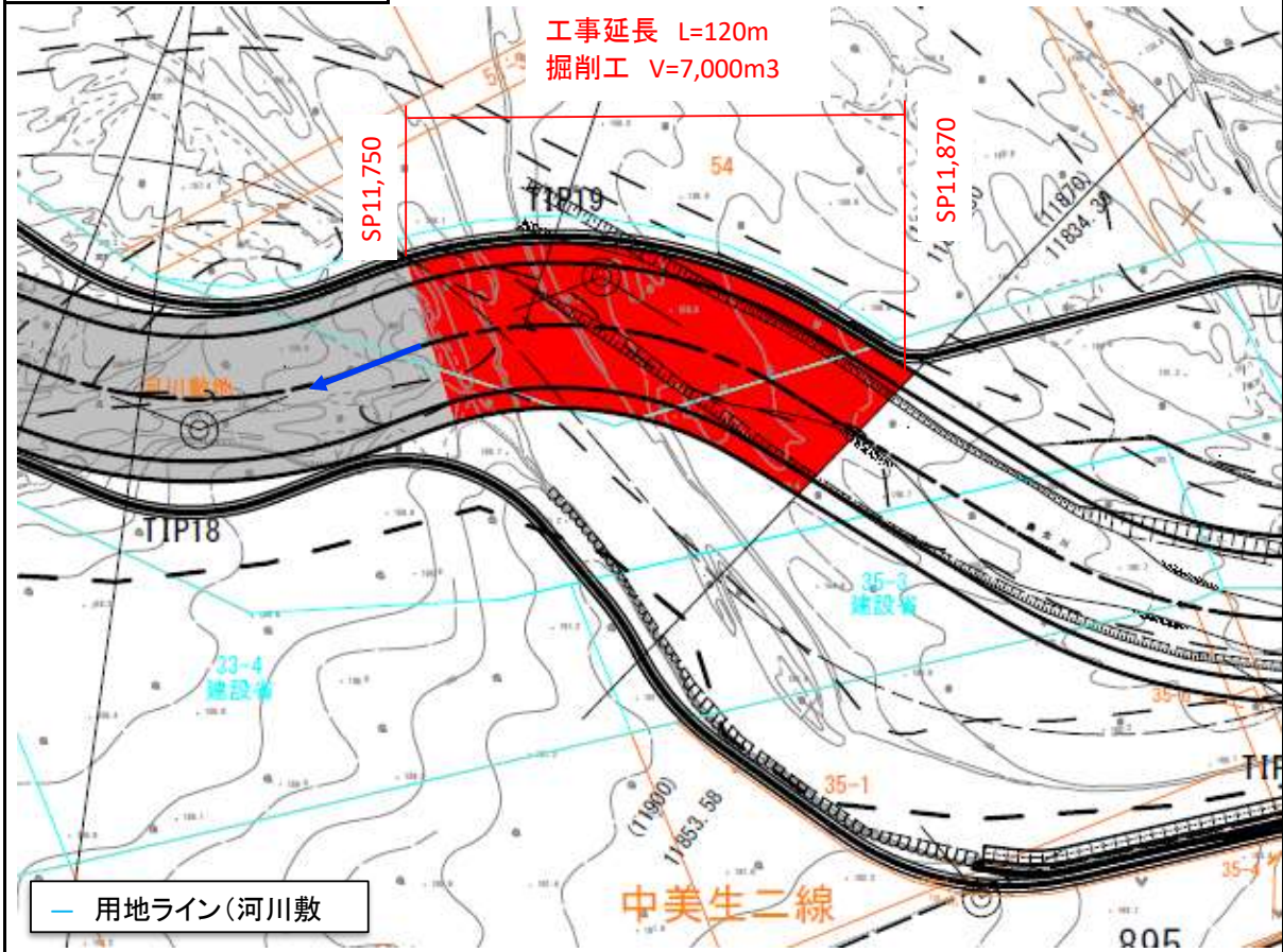
平 面 図
