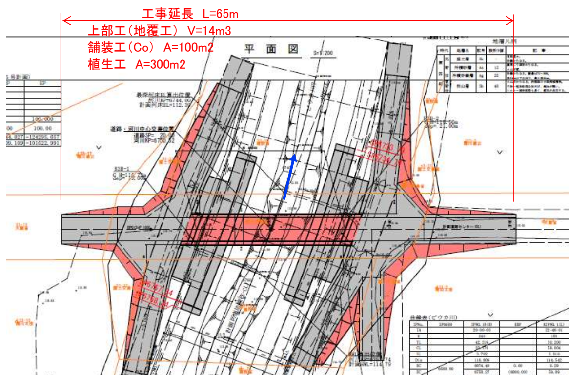
平 面 四
